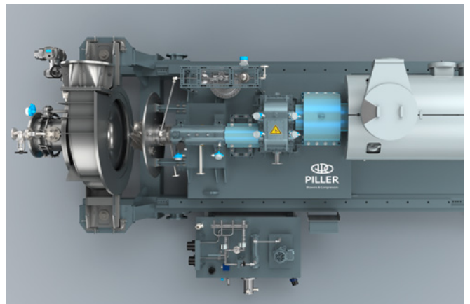
转子抽芯设计，便于维护和保养
