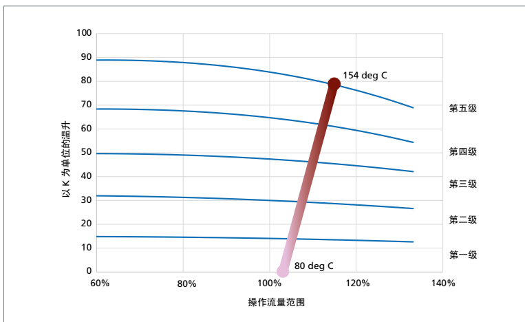
多级设计 - VapoMaxX 在压缩系统 1 中的性能
