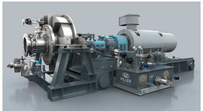
VapoMaxX – 先进的蒸汽压缩系统
