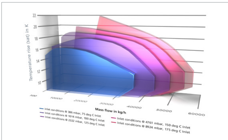
单级设计 - VapoMaxX 产品系列的性能总结
