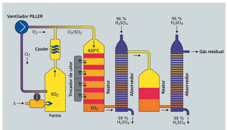
Esquema do processo de dupla absorção de contato
